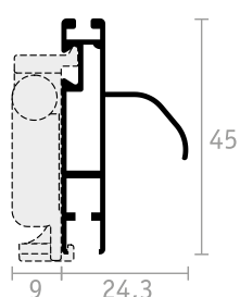
BARRA MANIGLIA
