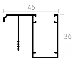
GUIDA
