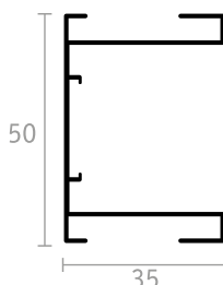
PROFILO INCASSO
