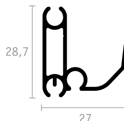
BARRA MANIGLIA
