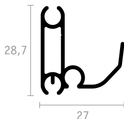
BARRA MANIGLIA
