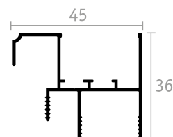
BATTUTA
