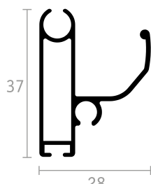
BARRA MANIGLIA
