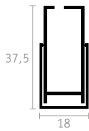
GUIDA TELESCOPICA
