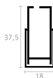
GUIDA SUPERIORE
