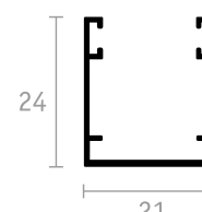
GUIDA INFERIORE
