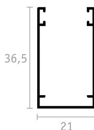
GUIDA SUPERIORE
