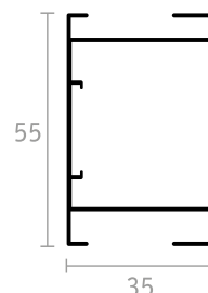
PROFILO INCASSO
