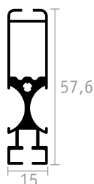
BARRA MANIGLIA
