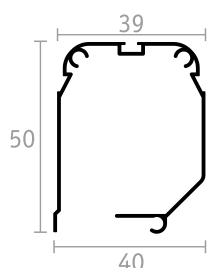
CASSONETTO
