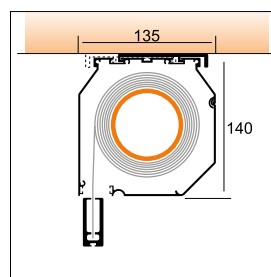
Ingombri
