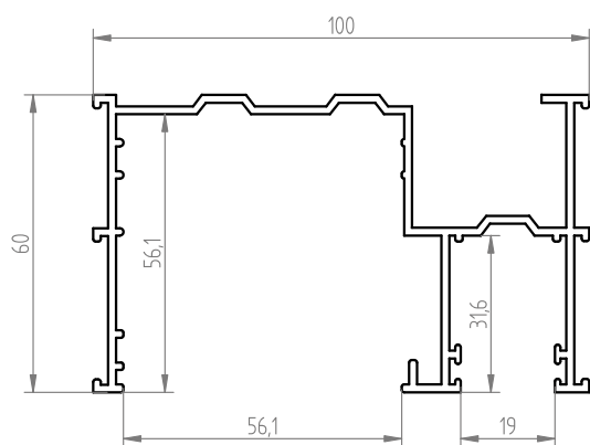
1A00332xx_Profilo incasso 55 con guida avvolgibile
