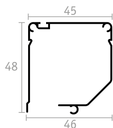
CASSONETTO
