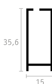
GUIDA SUPERIORE
