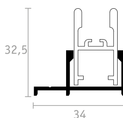
TELAIO 2 VIE CON COMPENSATORE
