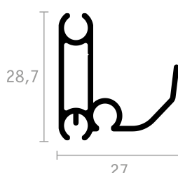
BARRA MANIGLIA
