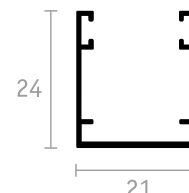
GUIDA INFERIORE
