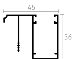
GUIDA SUPERIORE E BATTUTA
