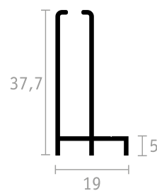
GUIDA AD L
