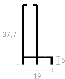
GUIDA AD L
