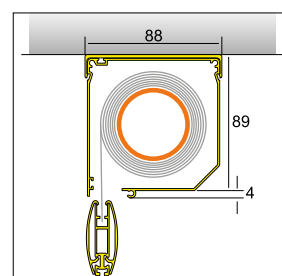
Ingombri
