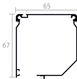
CASSONETTO 65
