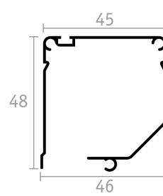
CASSONETTO 45
