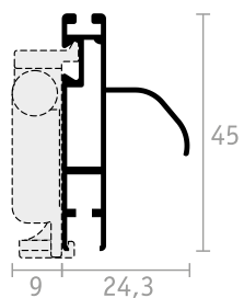
BARRA MANIGLIA
