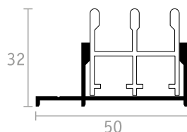
TELAIO CON COMPENSATORE
