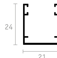
BATTUTA 21x24
