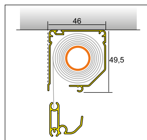
Ingombri
