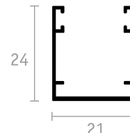
BATTUTA 21x24
