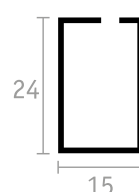
GUIDA INFERIORE
