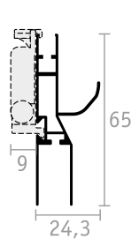
BARRA MANIGLIA SEMIFISSA
