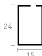
GUIDA INFERIORE
