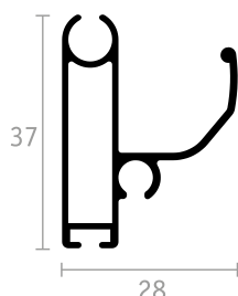
BARRA MANIGLIA
