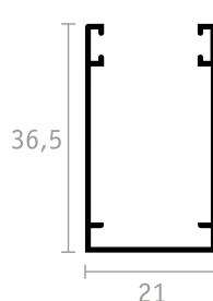
GUIDA SUPERIORE
