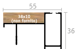
GUIDA SUPERIORE
