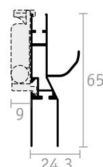
BARRA MANIGLIA (SEMIFISSA)
