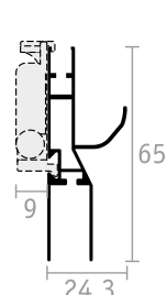
BARRA MANIGLIA (SEMIFISSA)
