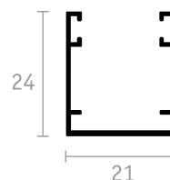
GUIDA INFERIORE E BATTUTA
