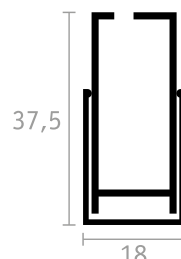
GUIDA SUPERIORE
