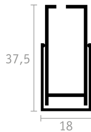
GUIDA TELESOPICA
