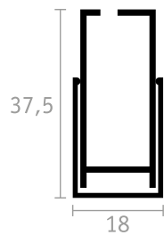
GUIDA TELESCOPICA
