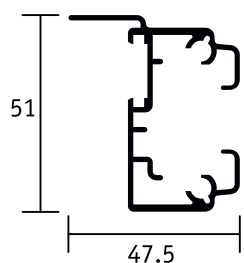
PROFILO MOBILE PER PACCO RUOTABILE
