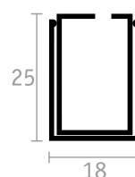
GUIDA INFERIORE
