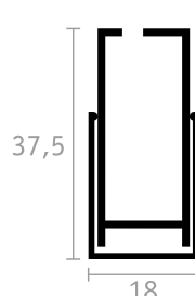
GUIDA SUPERIORE
