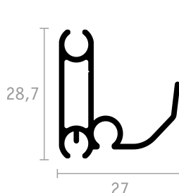
BARRA MANIGLIA
