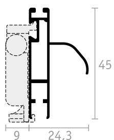
BARRA MANIGLIA (APRIBILE)
