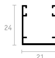
BATTUTA 21x24
