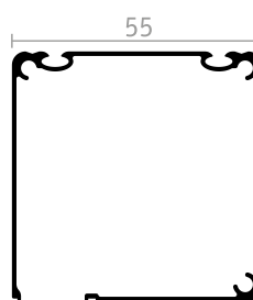
CASSONETTO 55 INCASSO
