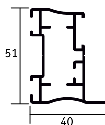
PROFILO A MURO PER PACCO RUOTABILE
