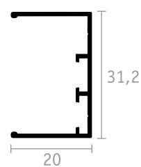
BATTUTA
