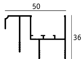
BATTUTA
