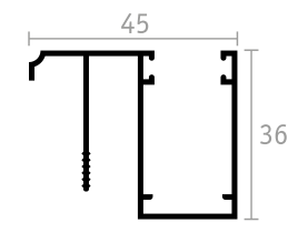
BATTUTA
