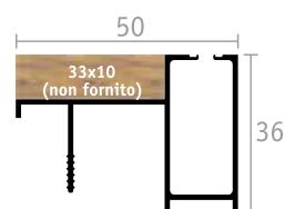
GUIDA
