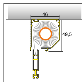
Ingombri
