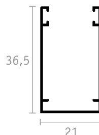
GUIDA SUPERIORE
