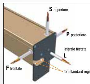
Tipologie uscita cavo motore e posizione registri
