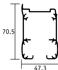
PORTA SERRATURA
