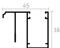
GUIDA SUPERIORE
