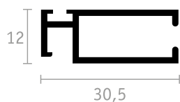
PROFILO PANNELLO
