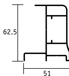
PROFILO PER MONTAGGIO OLTRE LUCE
