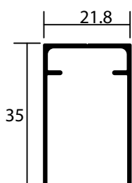
GUIDA SUPERIORE
