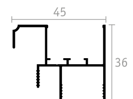
BATTUTA
