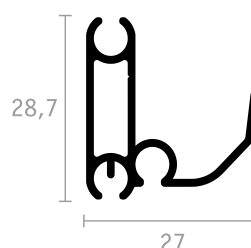
BARRA MANIGLIA
