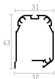
CASSONETTO
