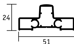
GUIDA INFERIORE
