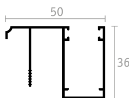
GUIDA SUPERIORE E BATTUTA
