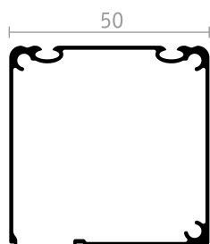
CASSONETTO 50 INCASSO
