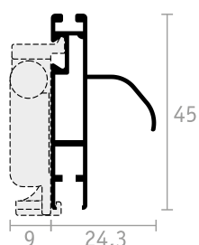
BARRA MANIGLIA (APRIBILE)
