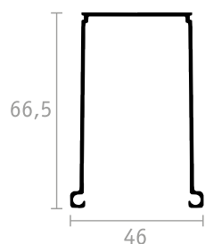
GUIDA SUPERIORE
