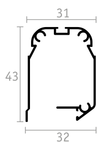
CASSONETTO
