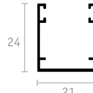
BATTUTA 21x24
