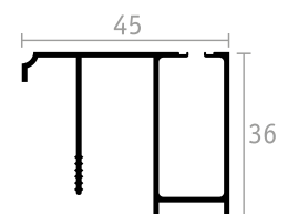
GUIDA SUPERIORE
