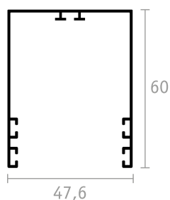
GUIDA SUPERIORE
