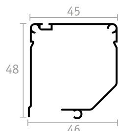
CASSONETTO
