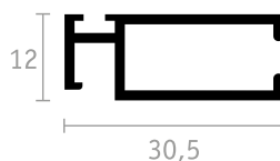
PORTARETE
