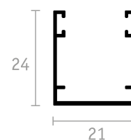
GUIDA INFERIORE
