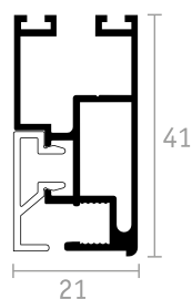
PROFILO PANNELLO
