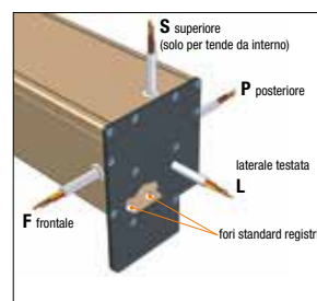
Uscite cavo motore e posizione registri
