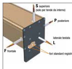
Tipologie uscita cavo motore e posizione registri
