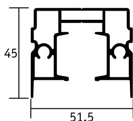
GUIDA SUPERIORE
