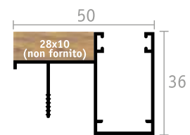
BATTUTA
