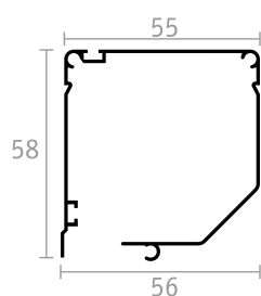
CASSONETTO 55
