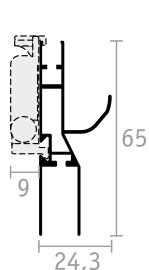
BARRA MANIGLIA SEMIFISSA
