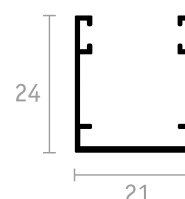
GUIDA INFERIORE
