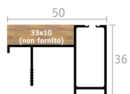
GUIDA
