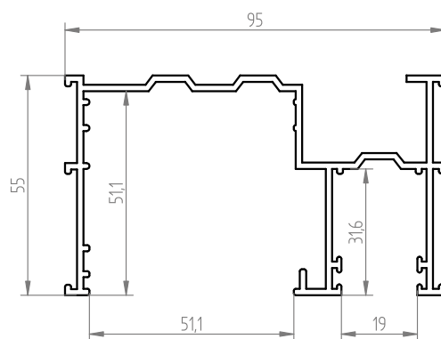
1A00330xx_Profilo incasso 50 con guida avvolgibile
