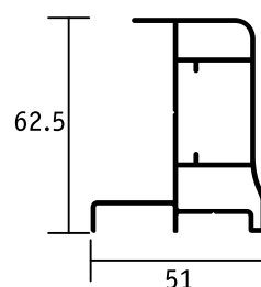
PROFILO PER MONTAGGIO OLTRE LUCE
