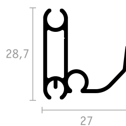
BARRA MANIGLIA
