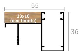
BATTUTA
