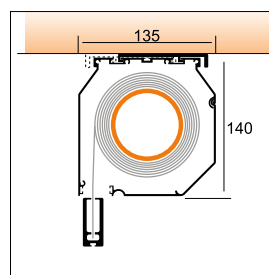
Ingombri
