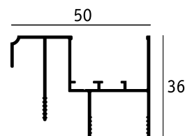
BATTUTA
