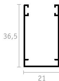
GUIDA SUPERIORE
