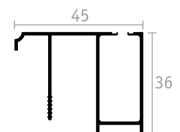
GUIDA SUPERIORE
