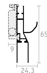
BARRA MANIGLIA (SEMIFISSA)
