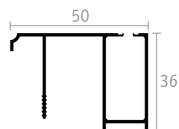
GUIDA SUPERIORE
