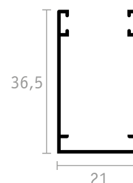
GUIDA
