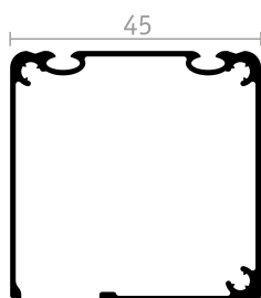
CASSONETTO
