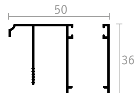
BATTUTA
