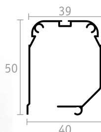
CASSONETTO
