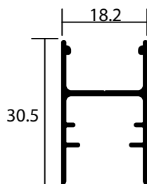
DORSO / CHIUSURA
