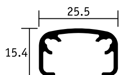
COPERTURA MONTANTI
