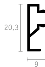
COPRIRETE
