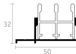
TELAIO 3 VIE CON COMPENSATORE
