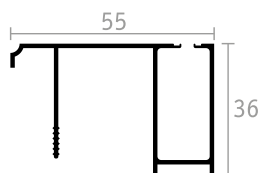
GUIDA SUPERIORE
