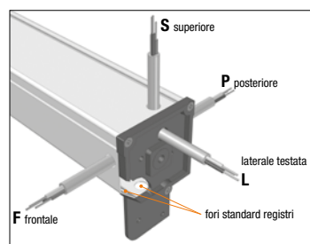
Tipologie uscita cavo motore e posizione registri
