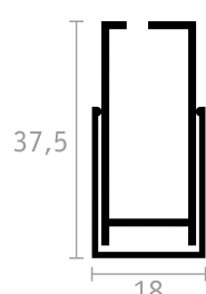
GUIDA TELESCOPICA SUPERIORE
