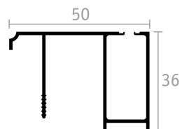
GUIDA SUPERIORE
