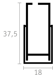
GUIDA TELESCOPICA
