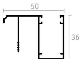
GUIDA SUPERIORE
