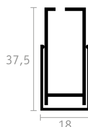
GUIDA SUPERIORE
