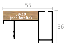
GUIDA SUPERIORE
