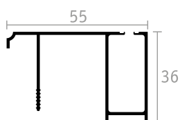
GUIDA SUPERIORE
