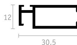
PROFILO PANNELLO
